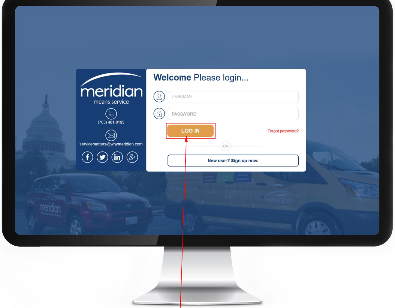
Login Button
